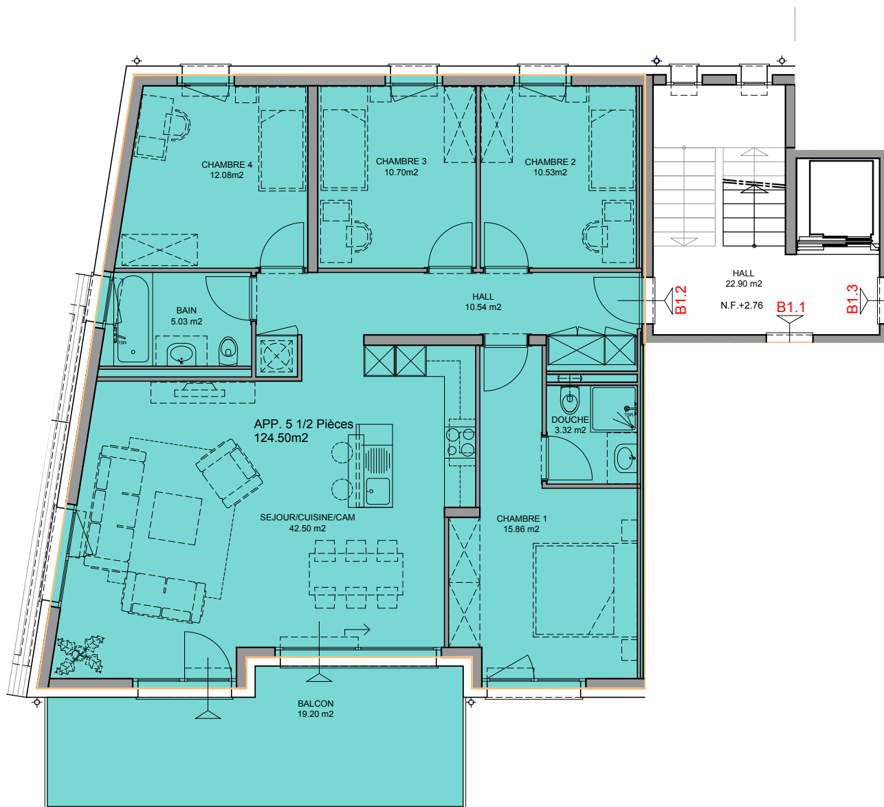
LOT B 1.2 - 5 1/2 Pièces 134.10 m 2 - Surface pondérée
